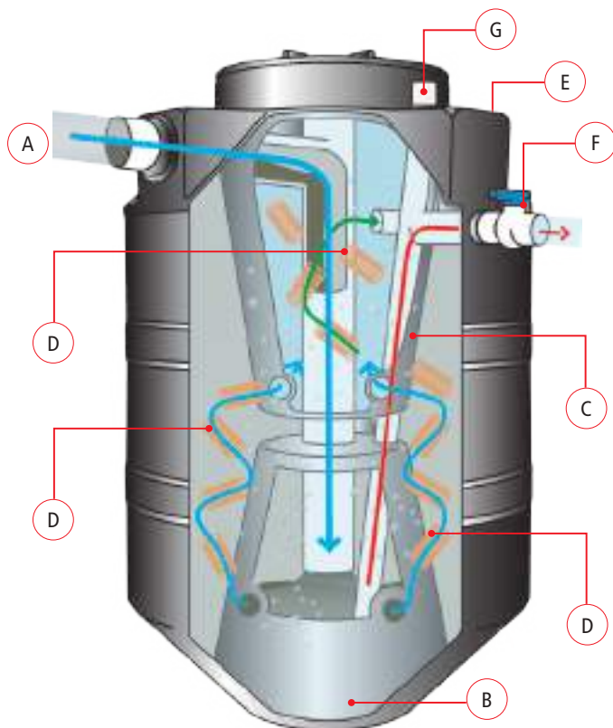
Funcionamiento - Acotaciones
